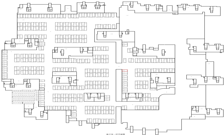
地下室一层平面图
